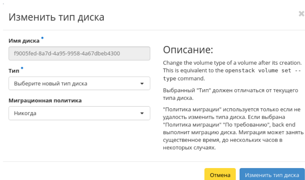
Рис. 3.85: Окно изменения типа диска
