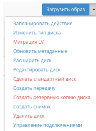
Рис. 3.75: Индивидуальные действия над диском
