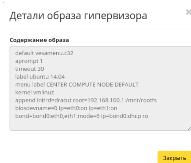
Рис. 3.188: Содержание образа гипервизора
