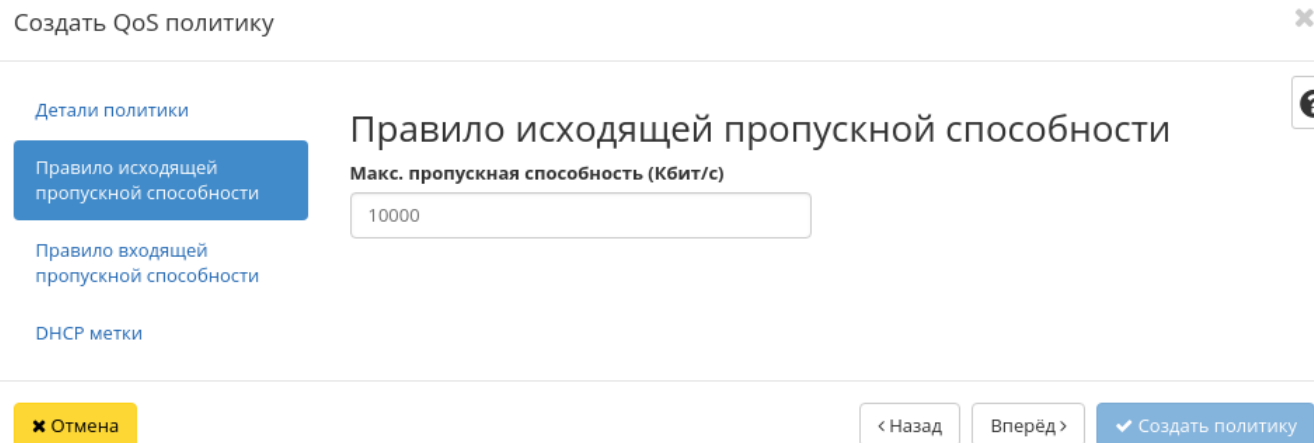
Рис. 3.138: Окно создания QoS политики
