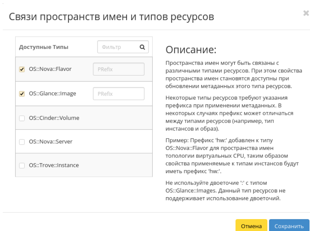
Рис. 4.303: Окно управления связями пространств имен и типов ресурсов
