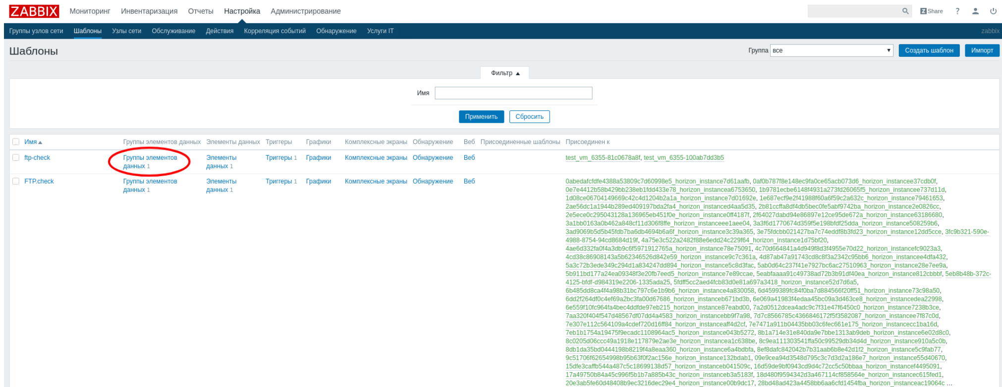
Рис. 4.6: Список шаблонов
