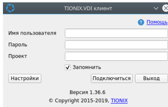
Рис. 6.20: TIONSIX.VDIclient
