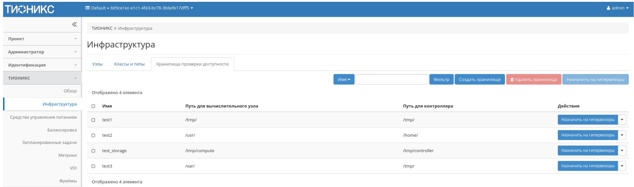
Рис. 3.395: Список хранилищ
