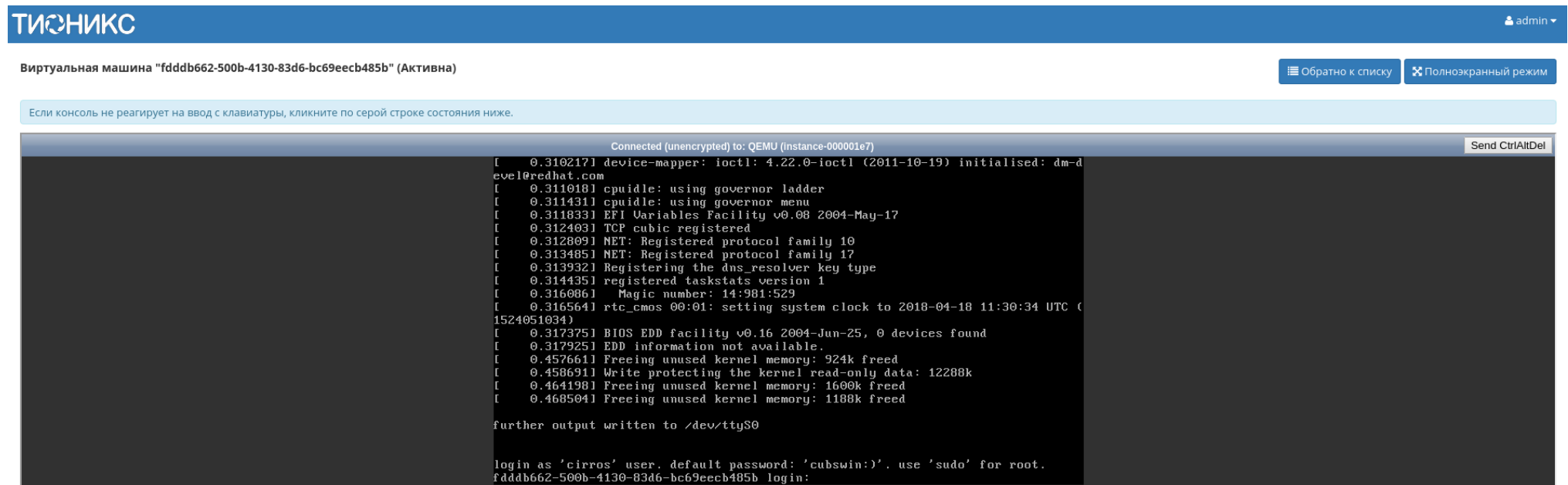
Рис. 3.517: Консоль машины
