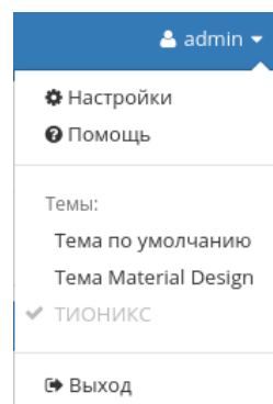
Рис. 3.521: Панель управления
