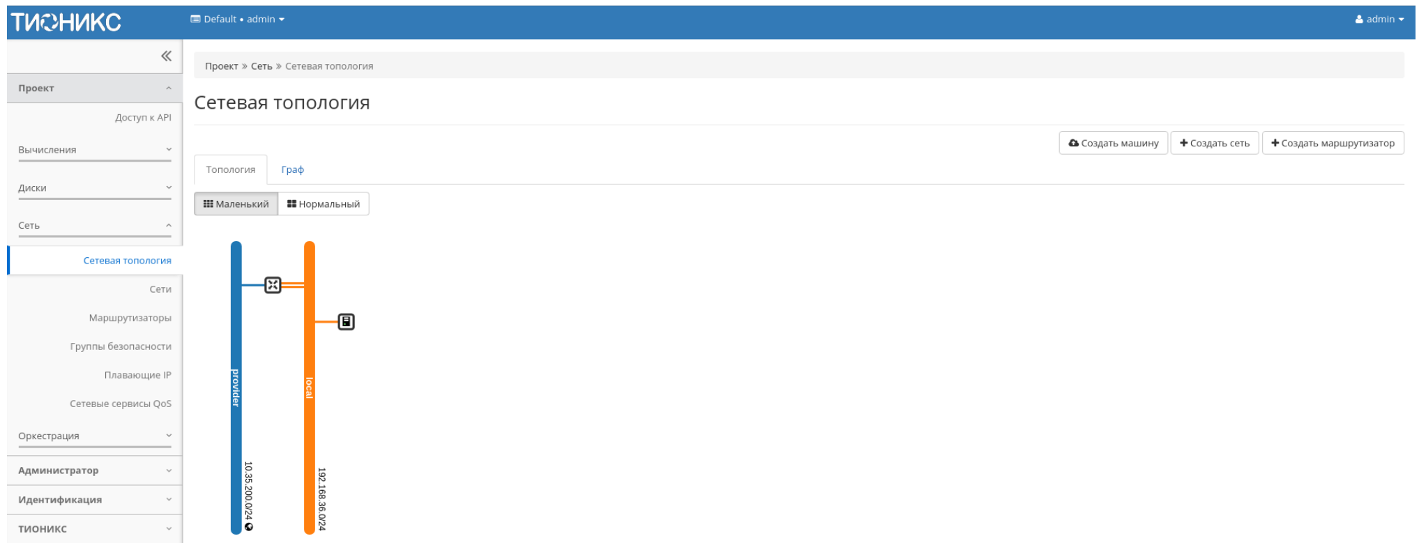
Рис. 3.104: Топология сети
