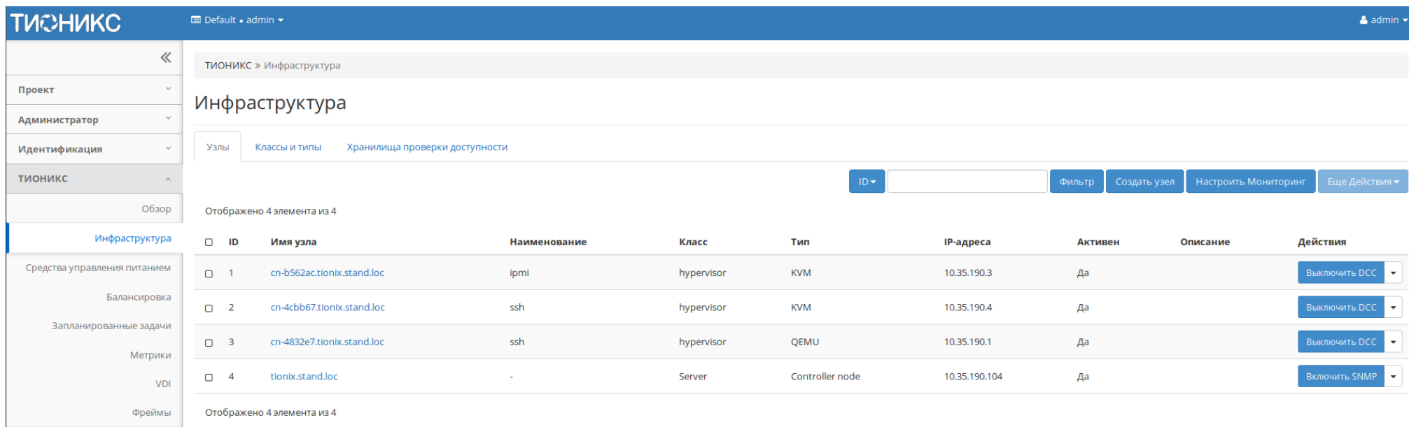
Рис. 3.373: Список узлов
