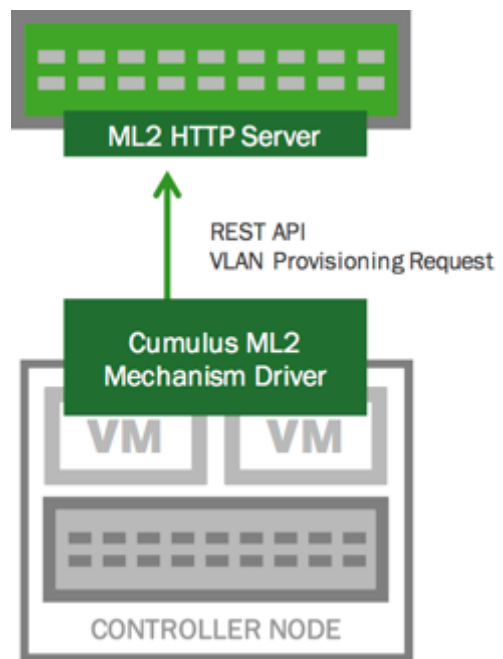
Рис. 10.1: Механизм ML2
