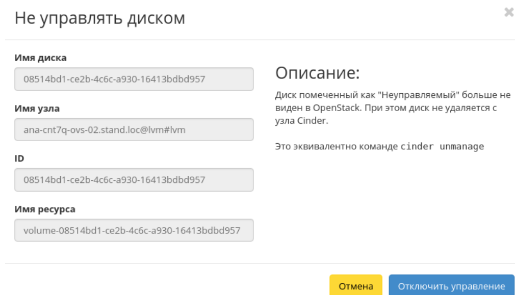
Рис. 3.255: Окно отключения возможности управления диском
