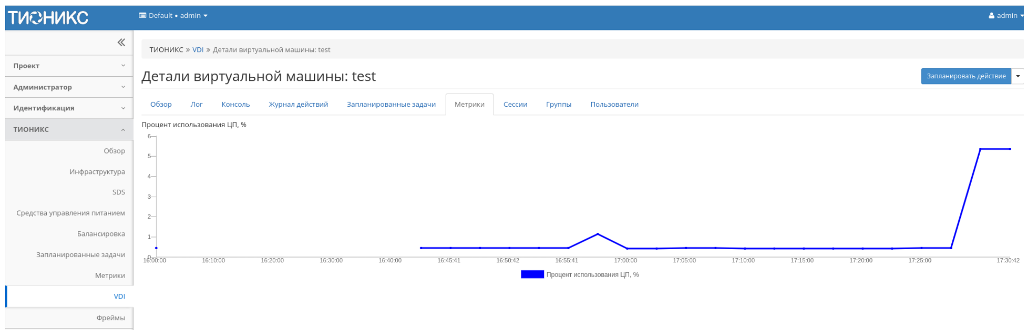
Рис. 3.458: Отображение статистики производительности VDI машины
