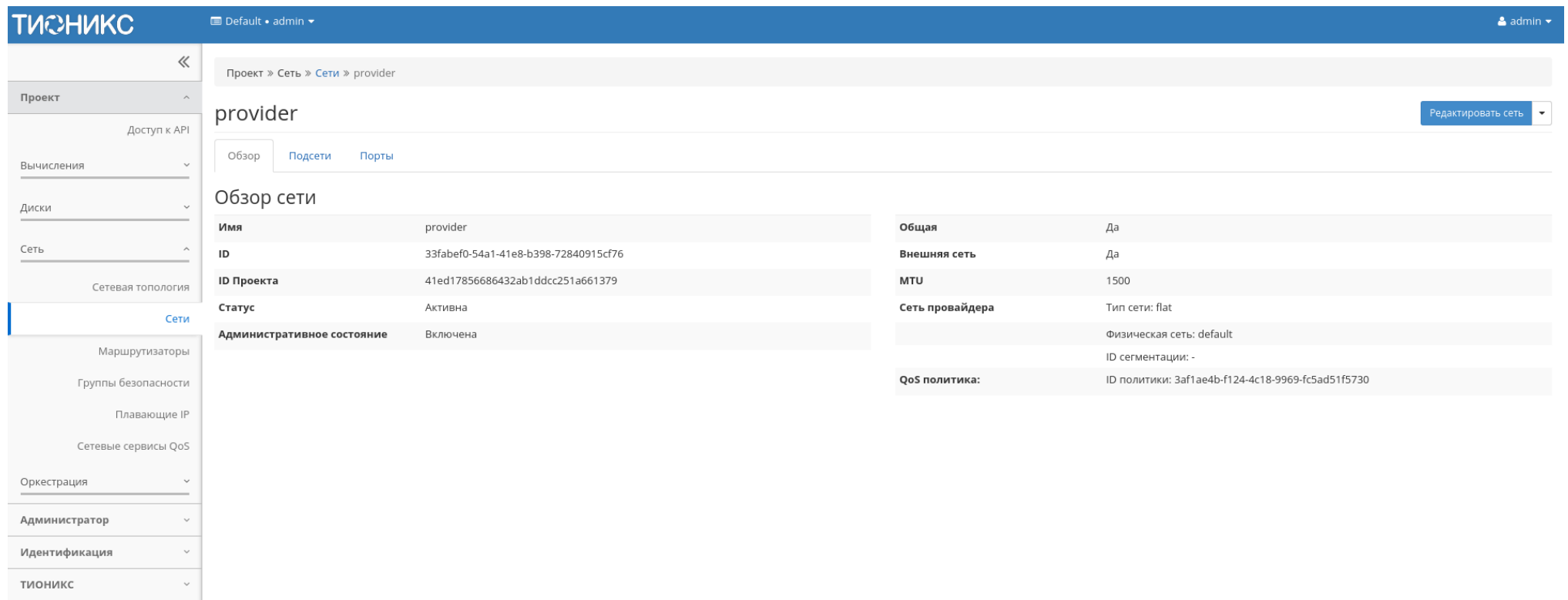
Рис. 4.107: Подробные параметры сети
