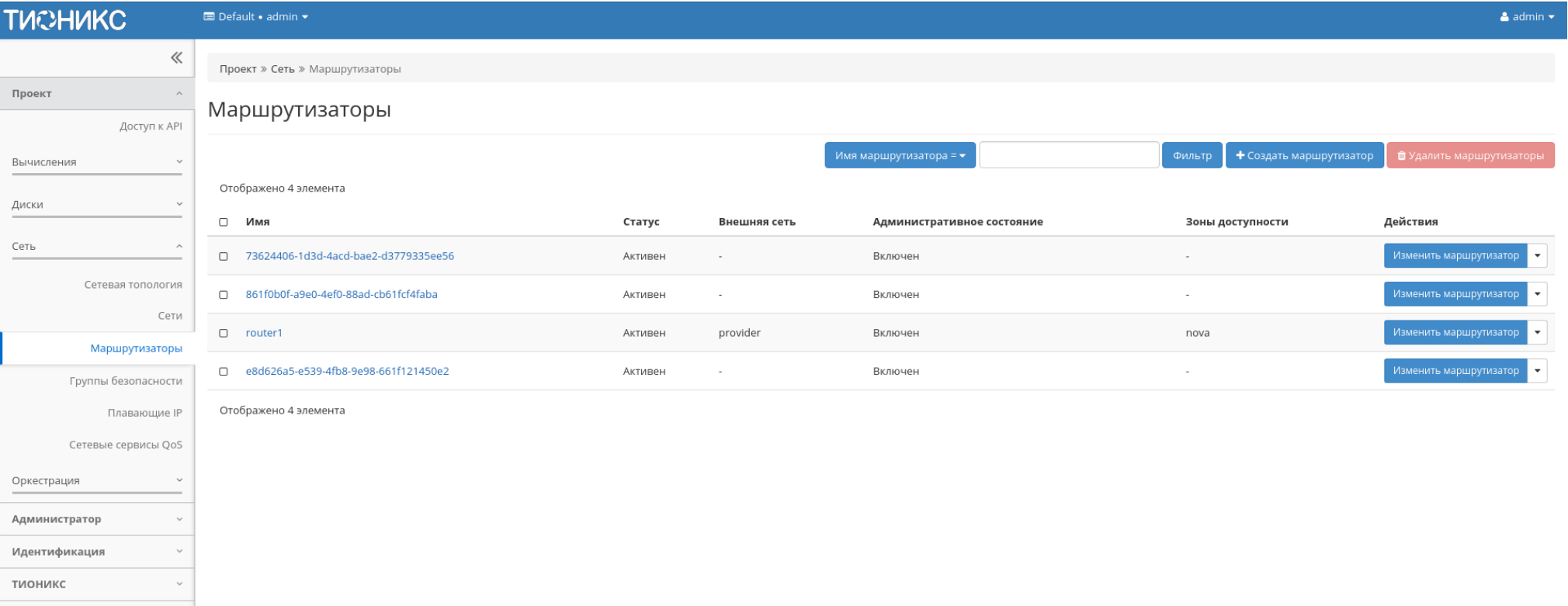
Рис. 4.119: Список маршрутизаторов
