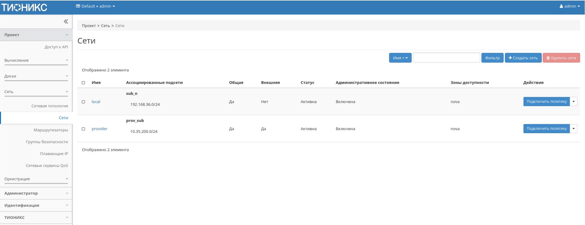
Рис. 4.106: Список сетей
