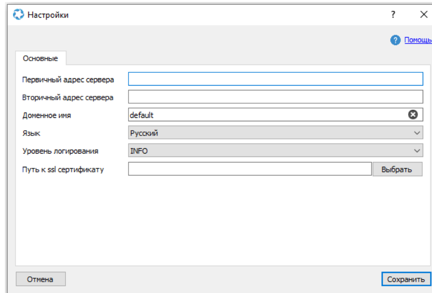
Рис. 6.20: Настройки
