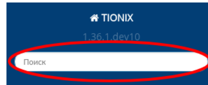
Рис. 14.1: Поисковая строка
