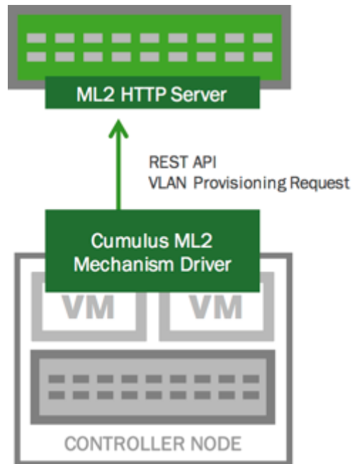
Рис. 9.1: Механизм ML2
