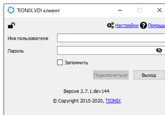
Рис. 6.21: TIONIX.VDIclient
