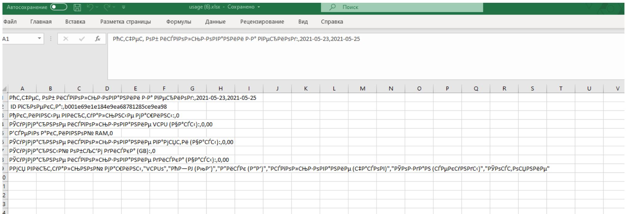
Рис. 14.3: Пример CSV-отчета
