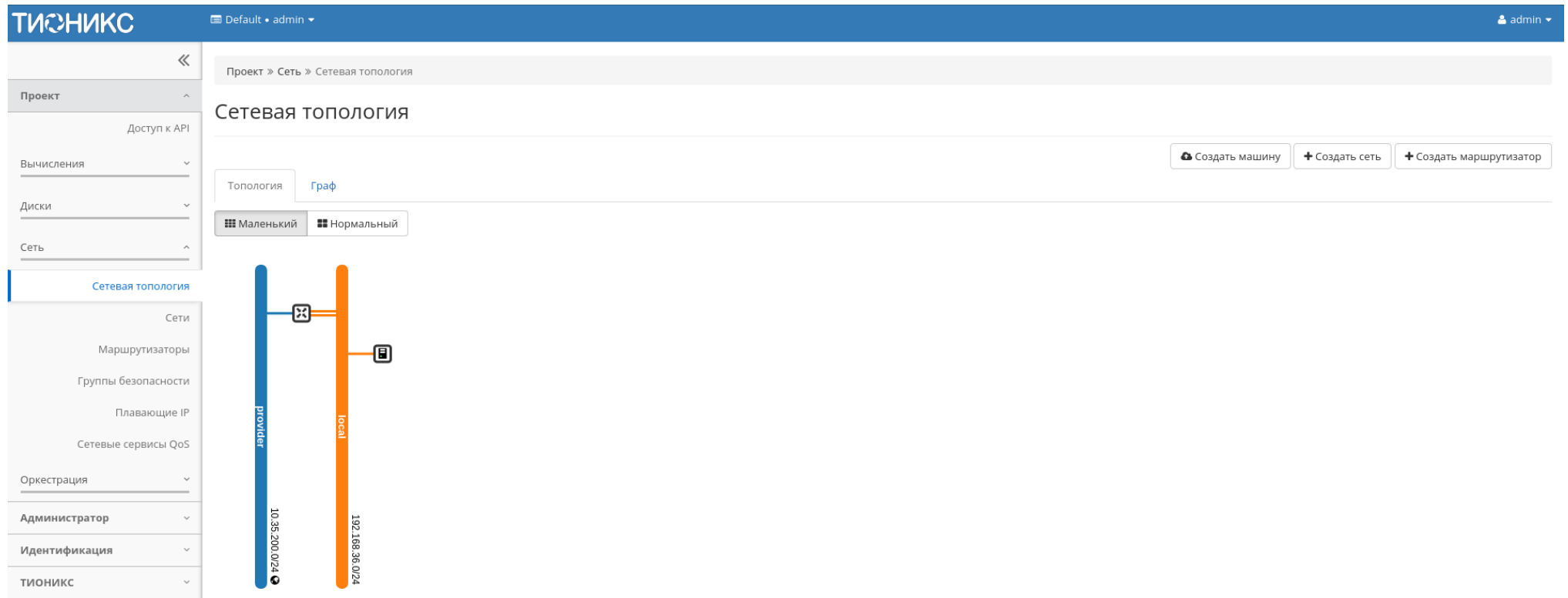
Рис. 3.104: Топология сети
