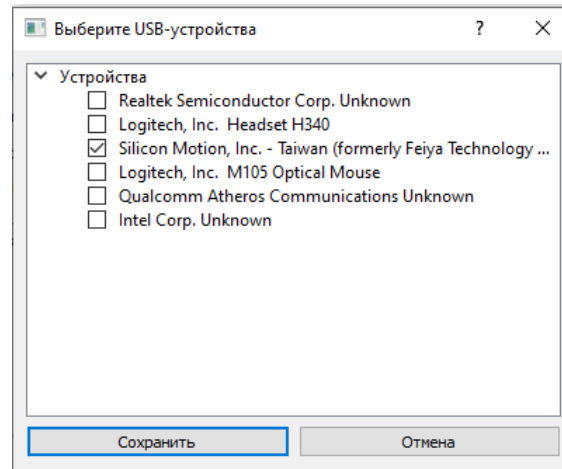
Рис. 6.31: Выбор USB-устройства
