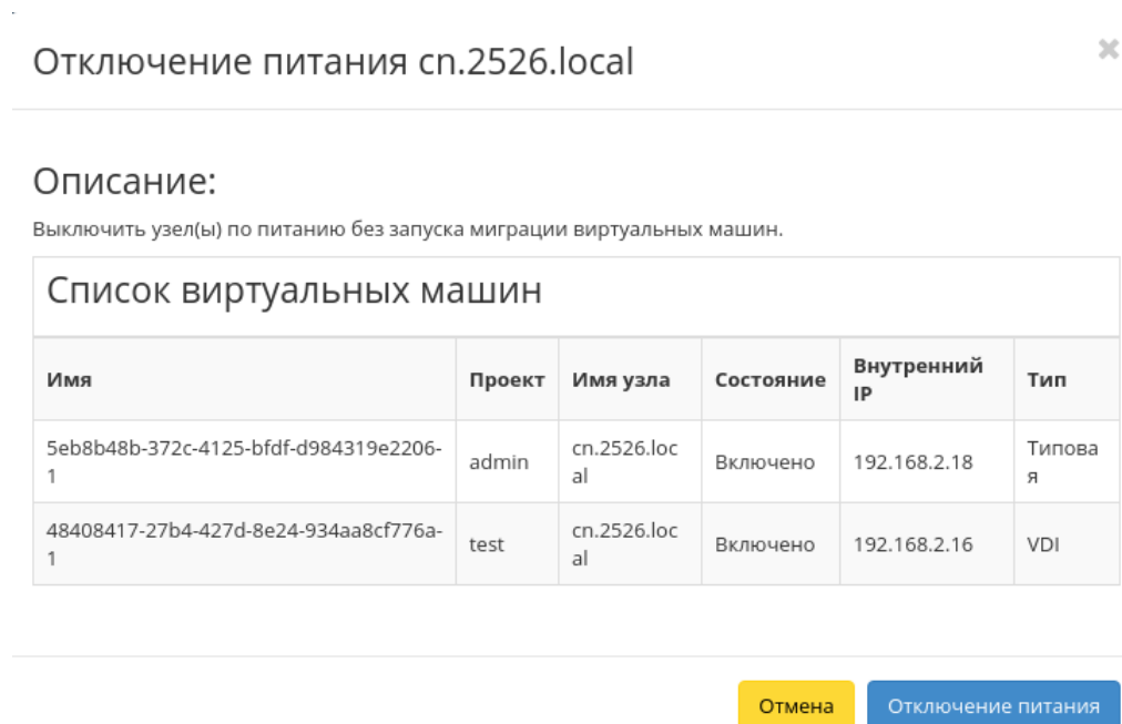
Рис. 4.178: Окно отключения питания гипервизора
