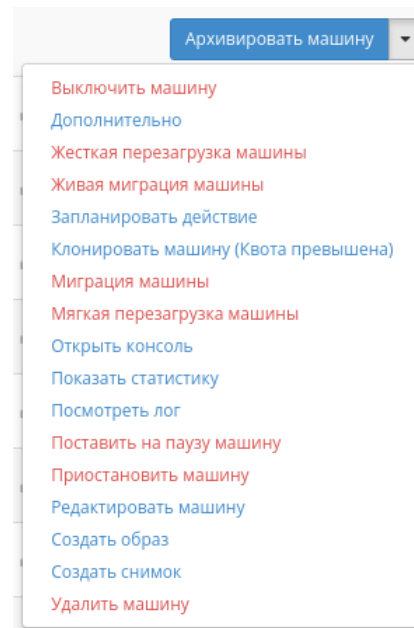
Рис. 4.213: Индивидуальные действия над виртуальной машиной
