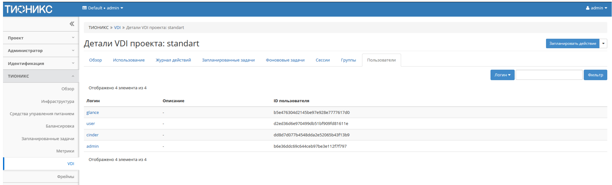
Рис. 4.503: Список пользователей VDI проекта
