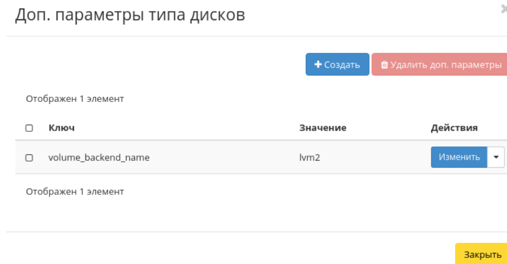
Рис. 4.277: Окно дополнительных параметров типа дисков
