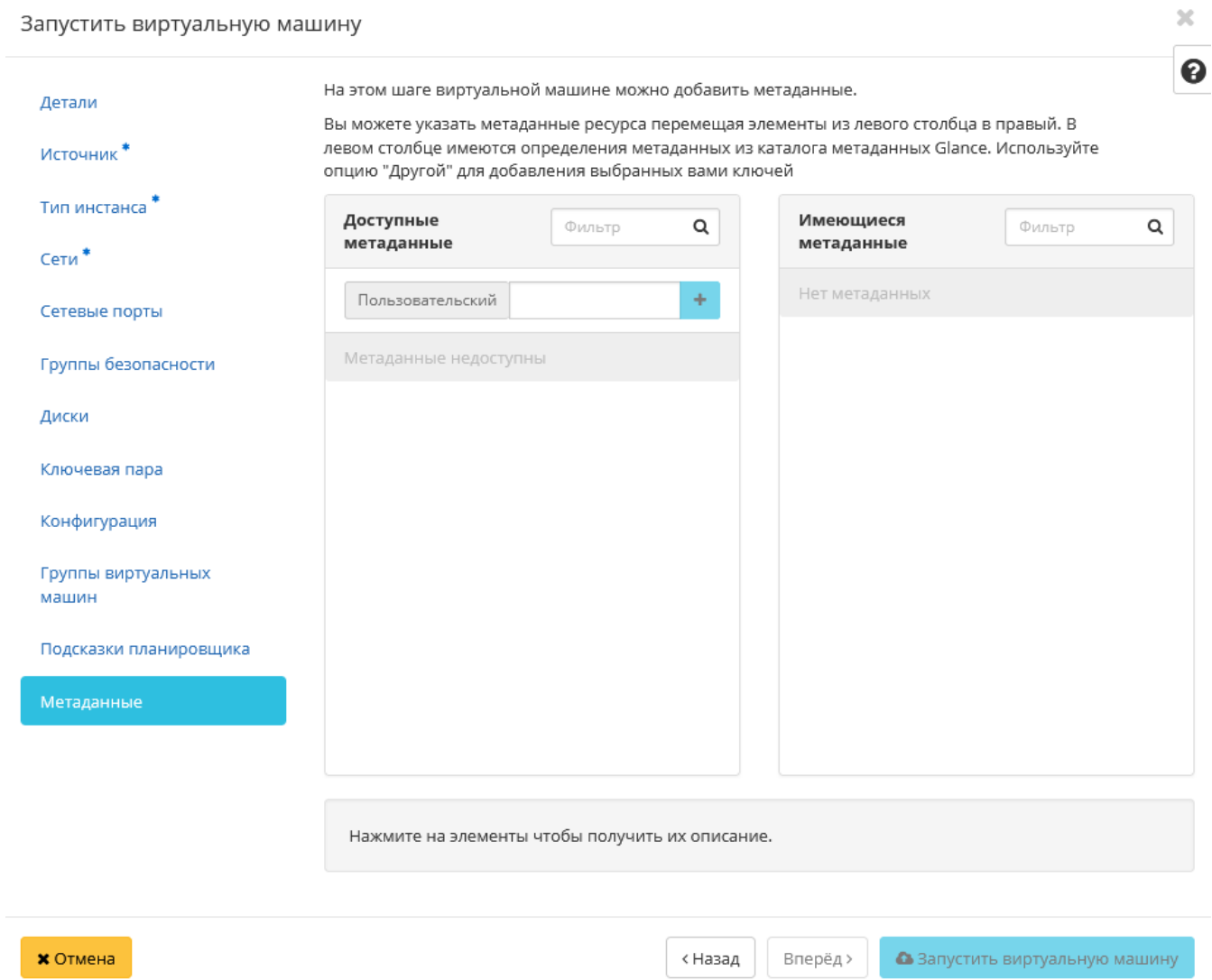
Рис. 4.37: Окно создания виртуальной машины
