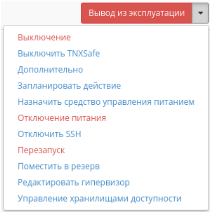
Рис. 4.170: Индивидуальные действия над гипервизором
