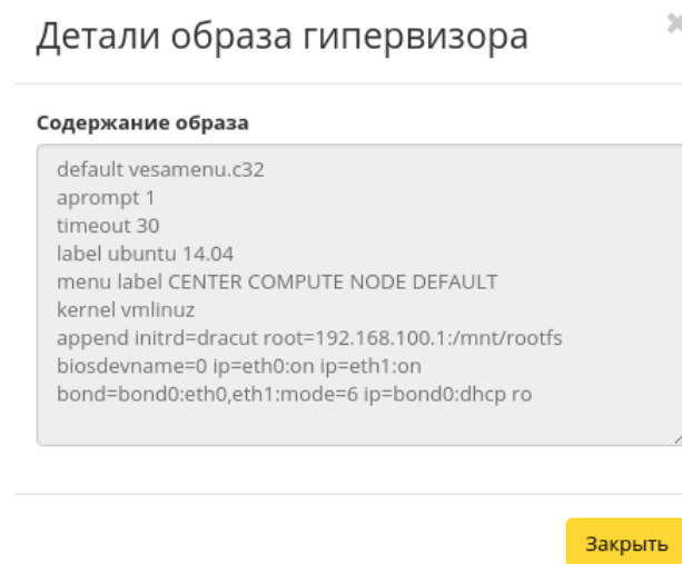
Рис. 4.196: Содержание образа гипервизора
