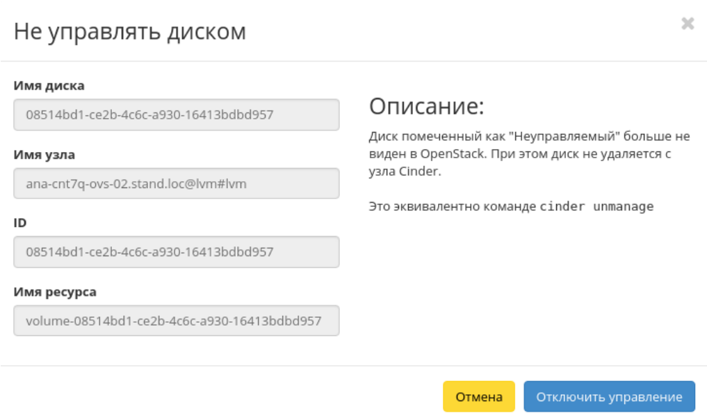
Рис. 4.263: Окно отключения возможности управления диском
