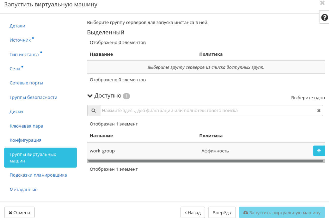
Рис. 4.35: Окно создания виртуальной машины
