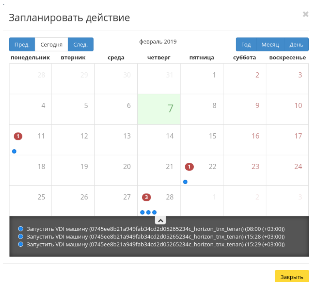
Рис. 4.491: Календарь планируемого действия
