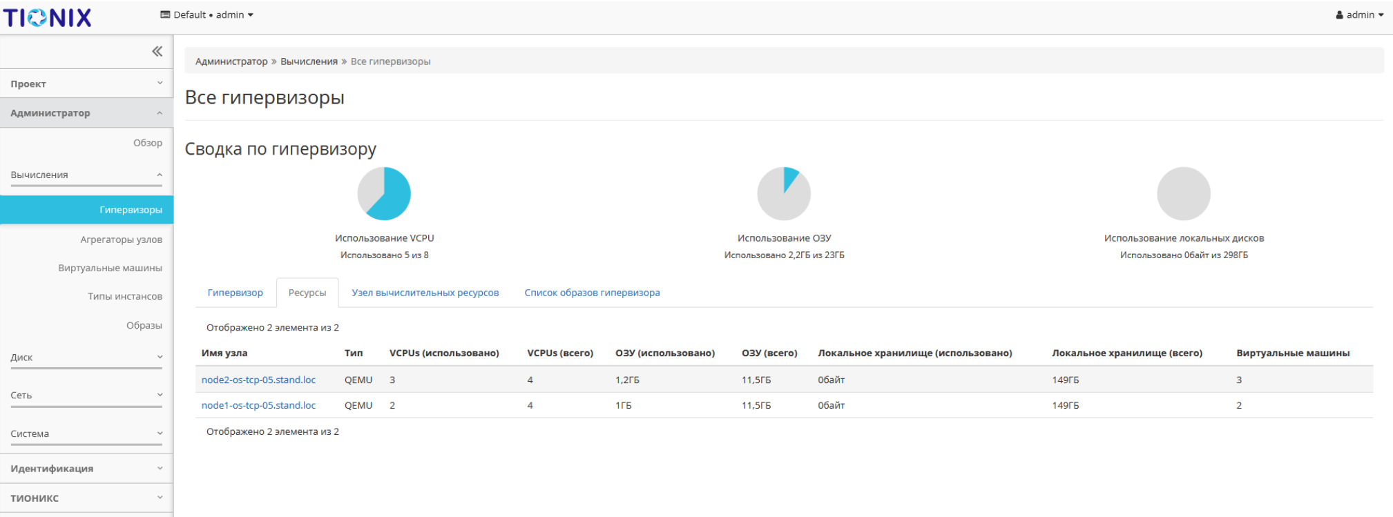
Рис. 4.157: Список гипервизоров
