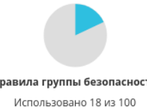
Рис. 4.3: Сводка лимитов
