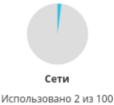
Рис. 4.3: Сводка лимитов
