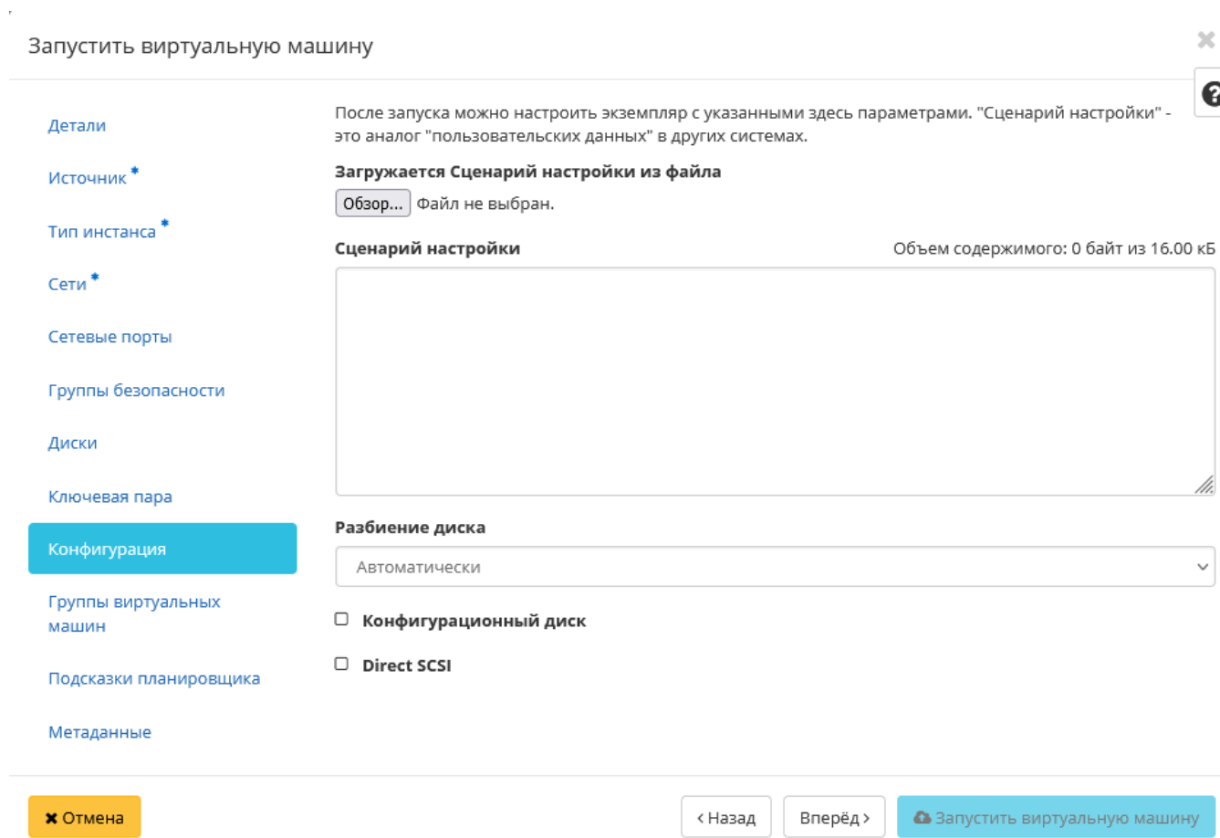
Рис. 4.32: Окно создания виртуальной машины
