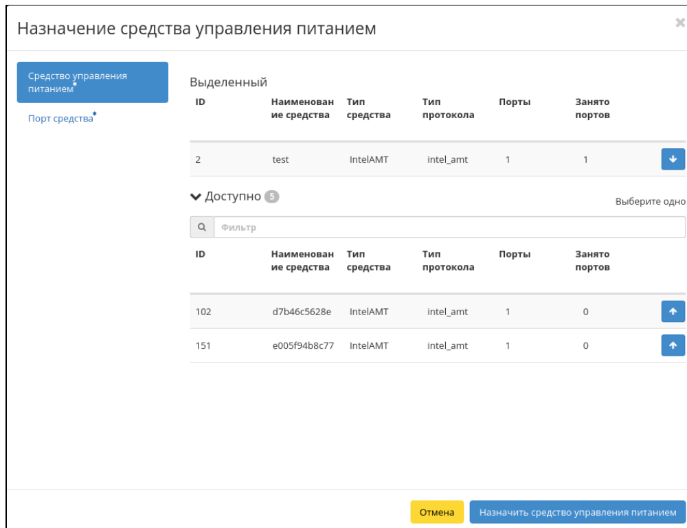
Окно назначения средства управления питанием гипервизору
