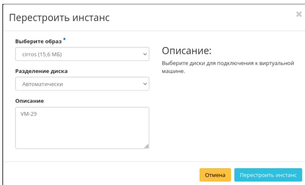
Окно перестройки машины
