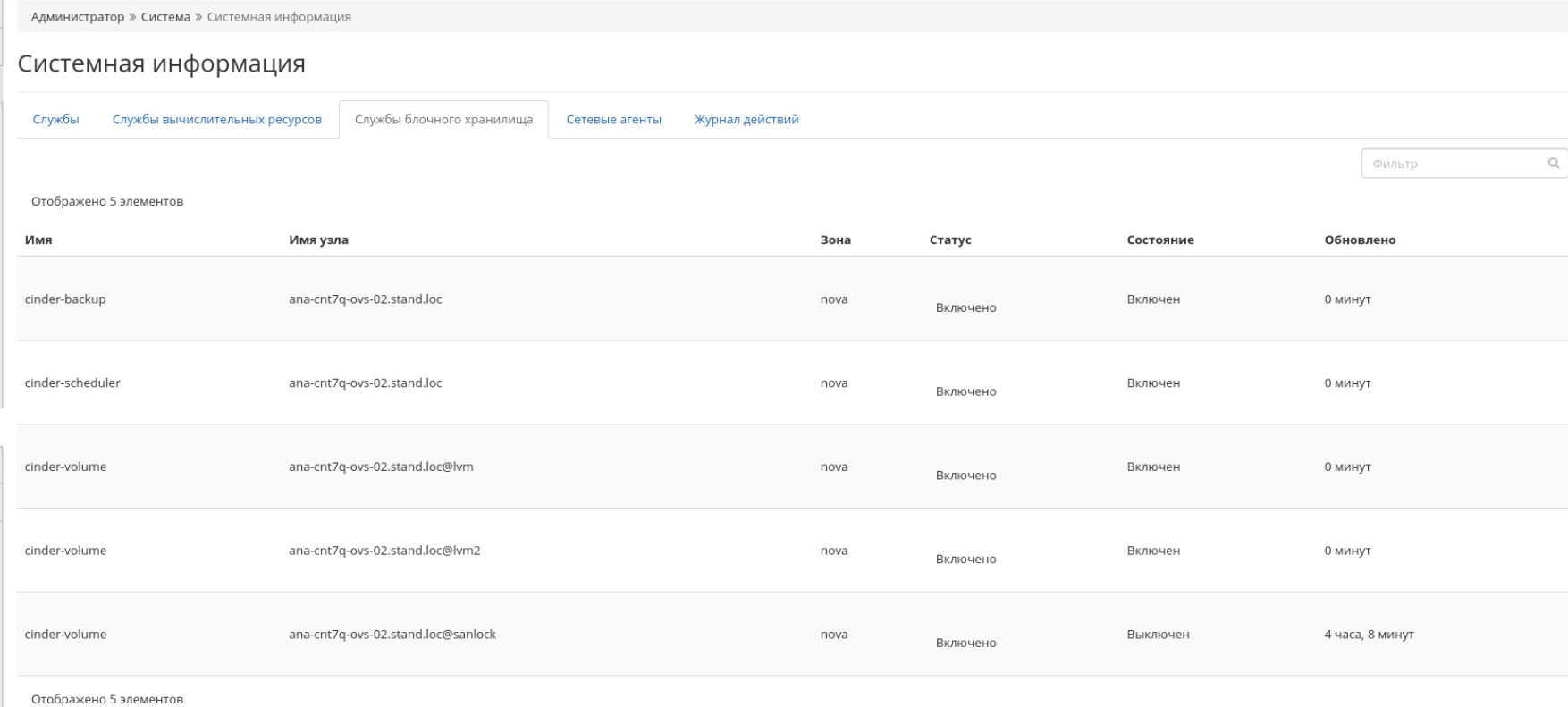
Рис. 4.322: Список служб блочного хранилища
