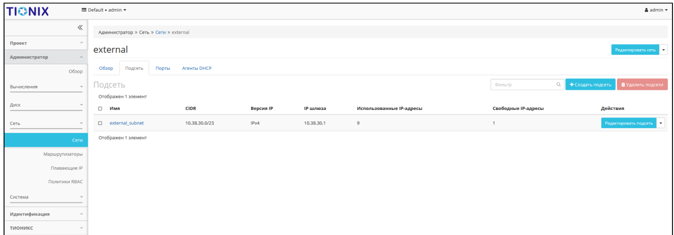
Список подсетей
