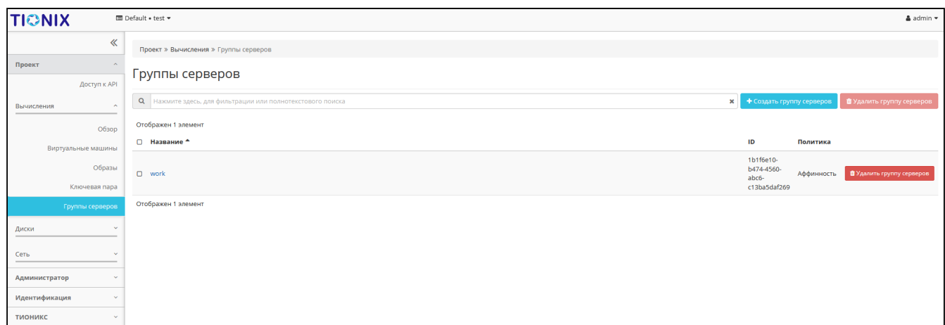
Список групп
