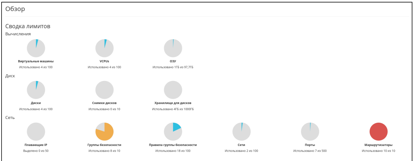
Сводка лимитов
