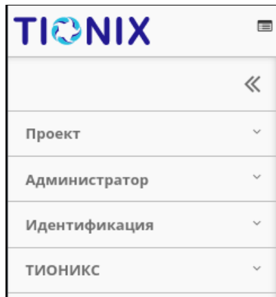
Панель навигации
