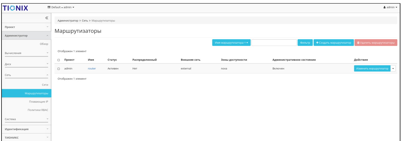
Список маршрутизаторов
