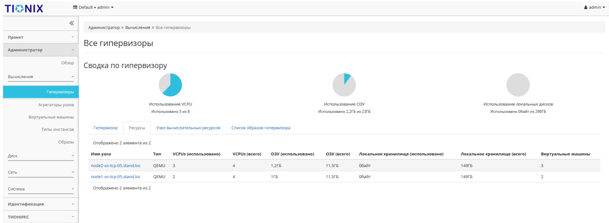
Рис. 4.157: Список гипервизоров
