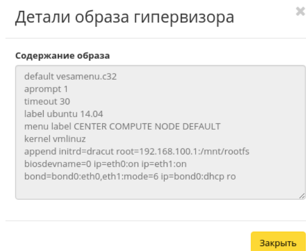
Рис. 4.194: Содержание образа гипервизора
