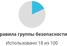
Рис. 4.3: Сводка лимитов
