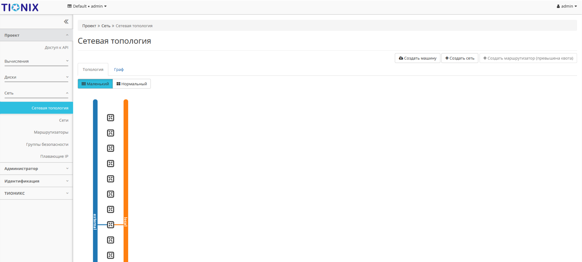
Рис. 4.110: Топология сети
