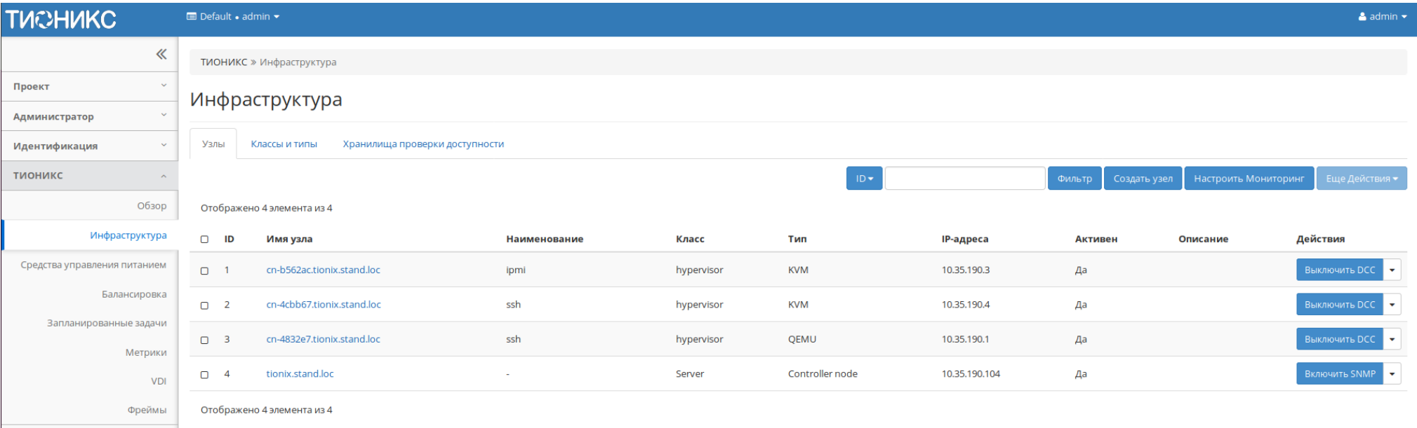
Рис. 4.395: Список узлов
