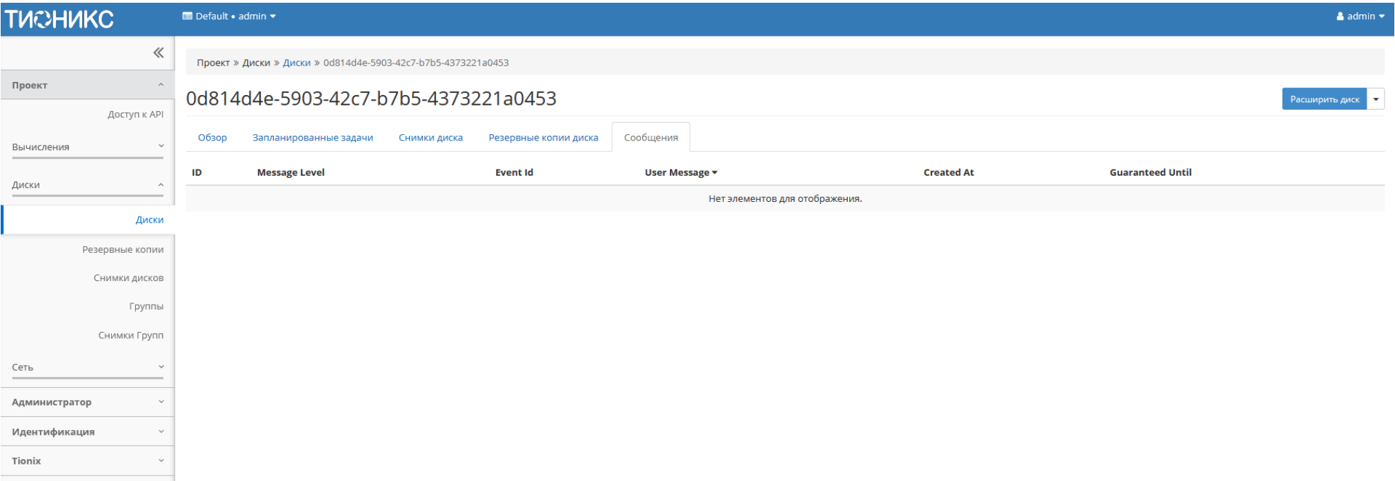
Рис. 4.76: Список сообщений
