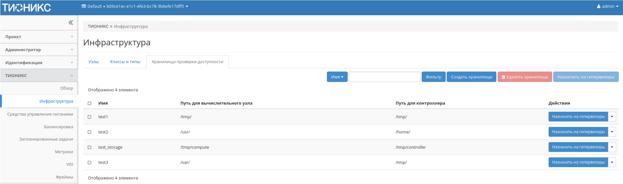
Рис. 4.417: Список хранилищ
