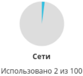
Рис. 4.3: Сводка лимитов
