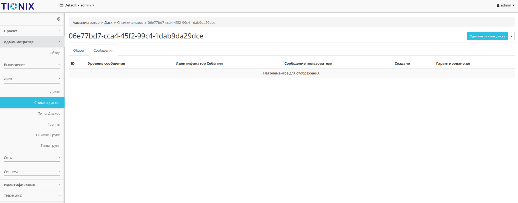
Рис. 4.265: Список сообщений
