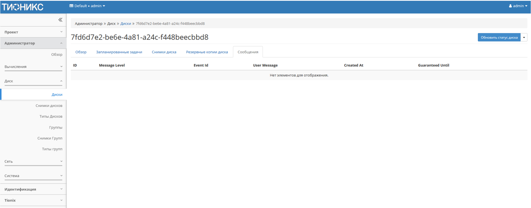
Рис. 4.248: Список сообщений
