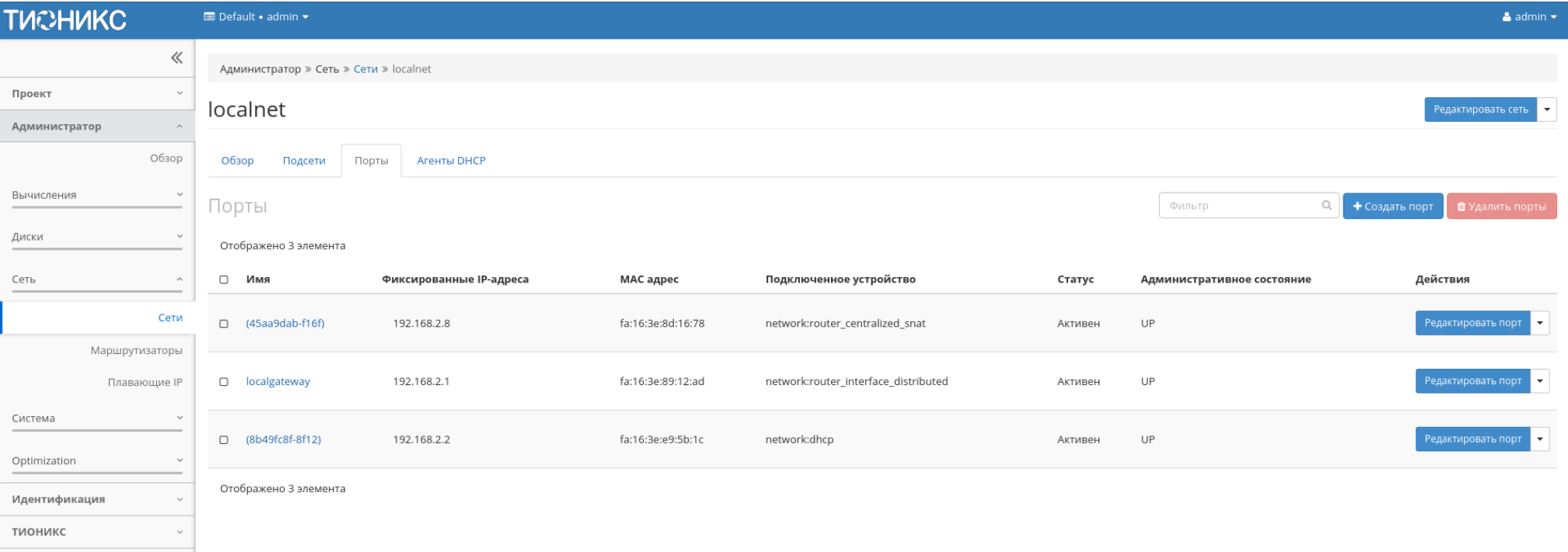
Рис. 4.288: Список портов
