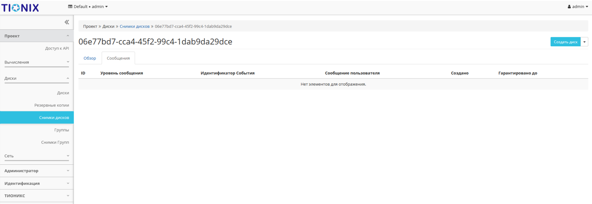
Рис. 4.102: Список сообщений
