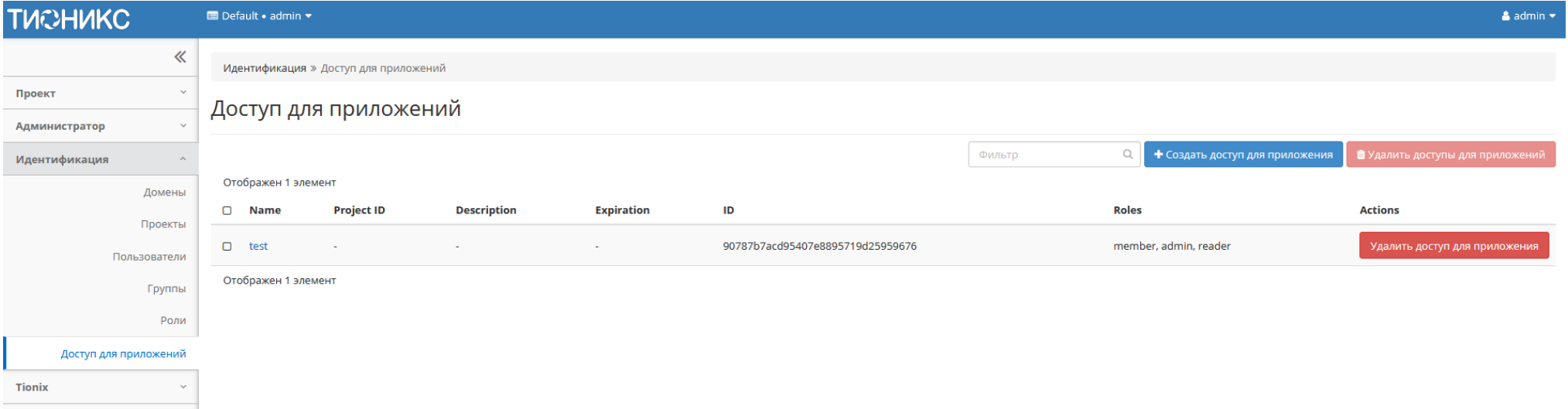
Рис. 4.387: Список приложений
