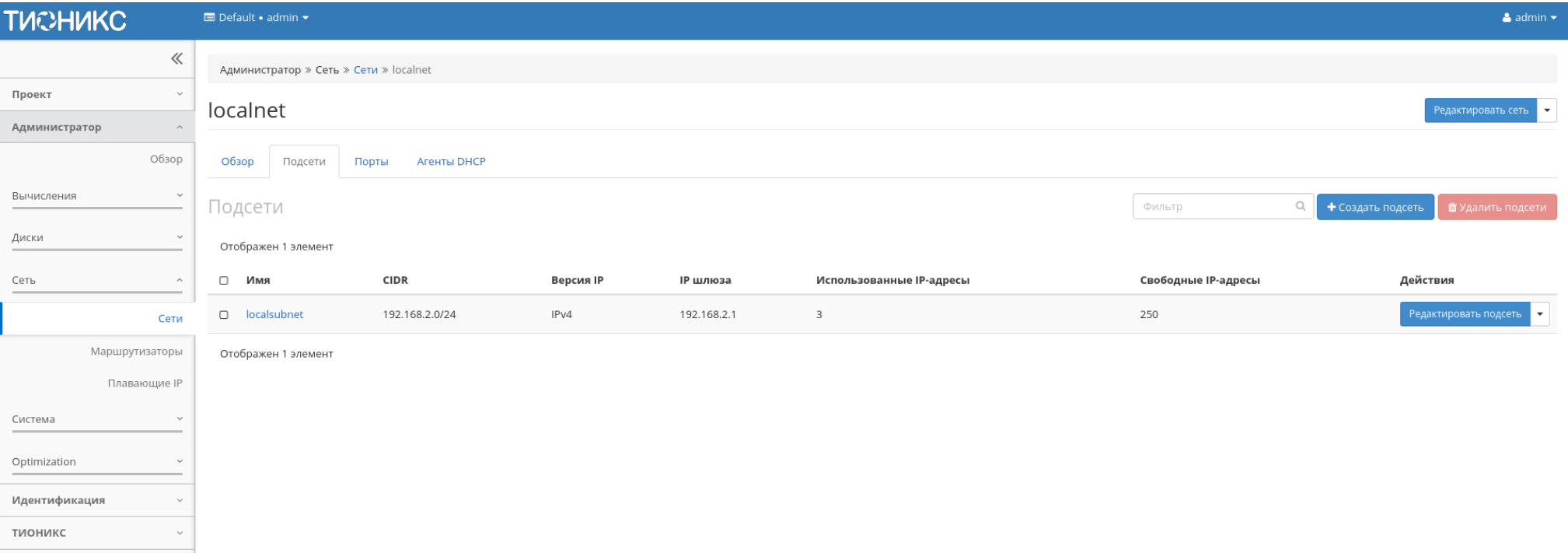
Рис. 4.287: Список подсетей
