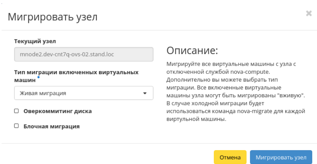
Рис. 4.187: Окно запуска миграции виртуальных машин с вычислительных узлов
