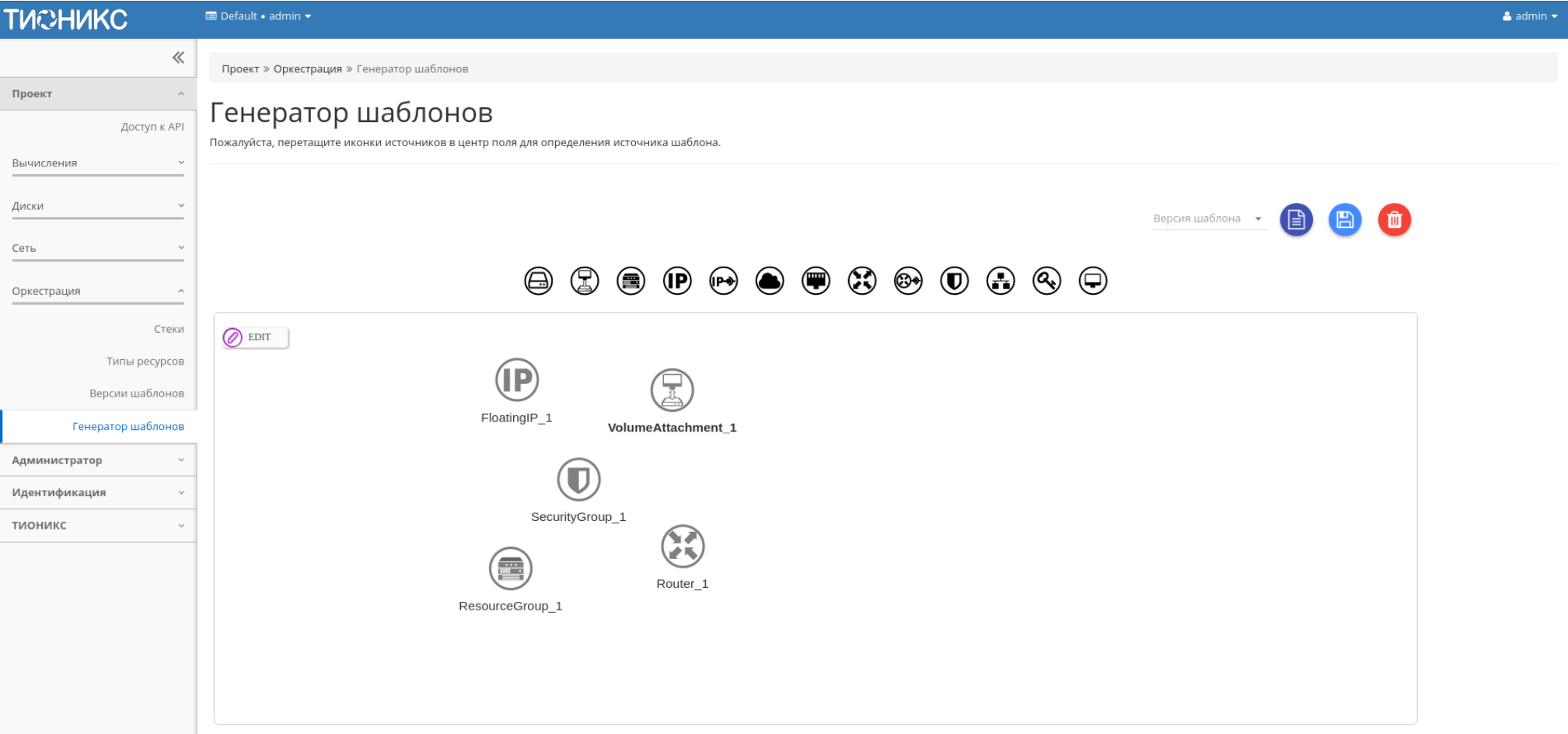
Рис. 4.154: Генератор шаблонов
