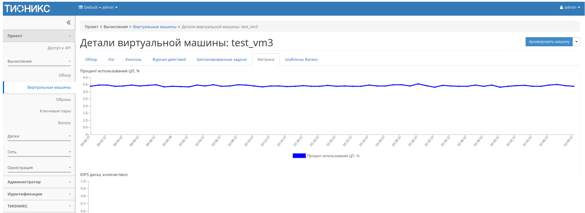
Рис. 4.32: Отображение статистики производительности виртуальной машины
