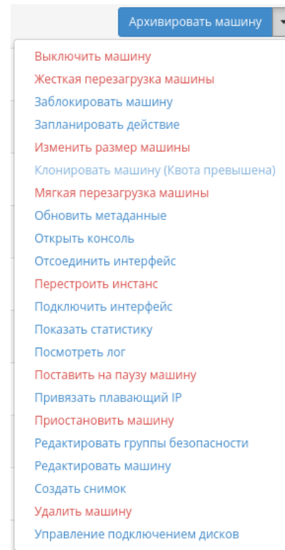
Рис. 4.35: Индивидуальные действия над виртуальной машиной
