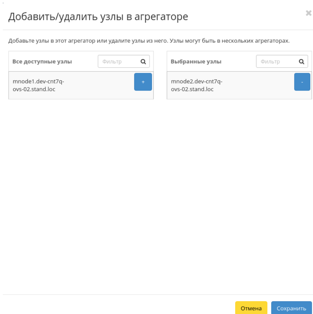
Рис. 4.221: Окно управления узлами
