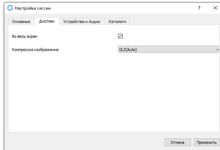
Рис. 3.101: Настройки дисплея VDI-сессии
