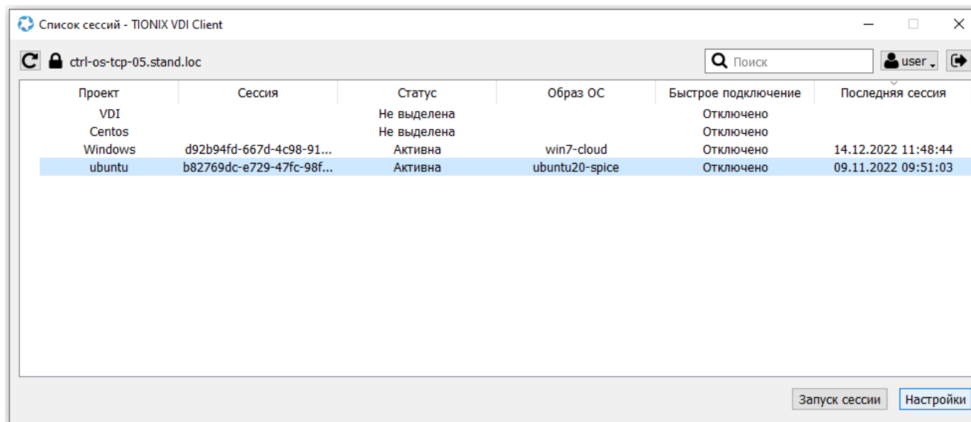
Рис. 3.98: Форма со списком VDI-сессий
