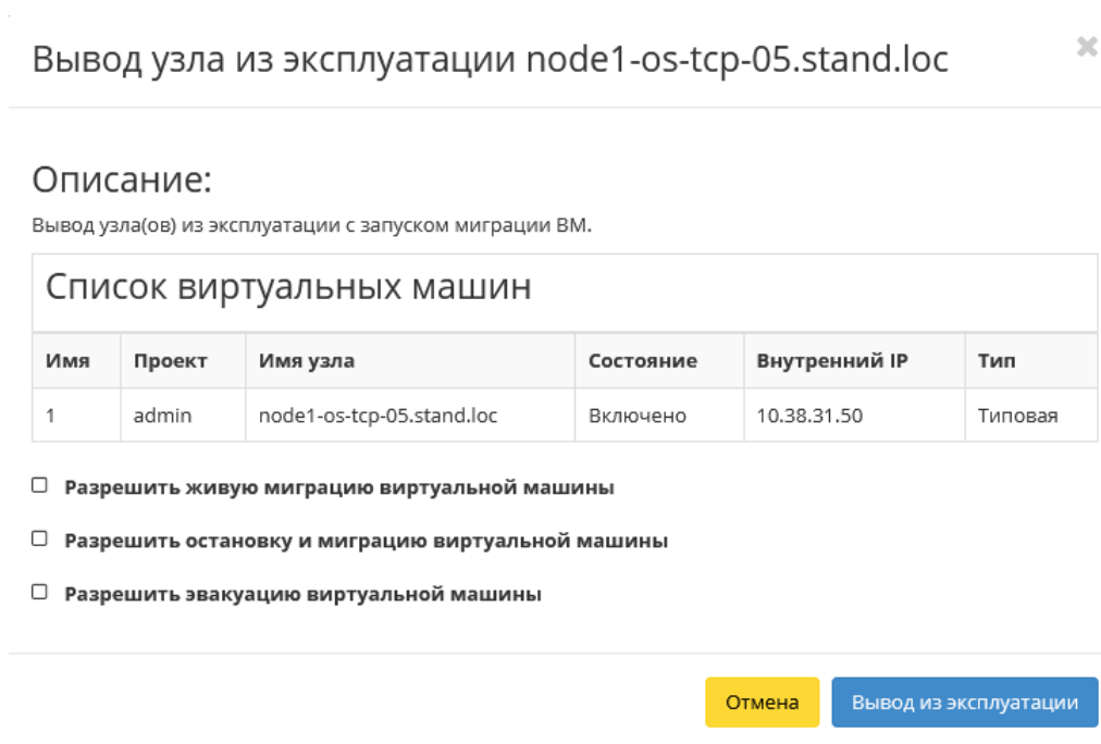
Рис. 4.197: Окно вывода гипервизора из эксплуатации
