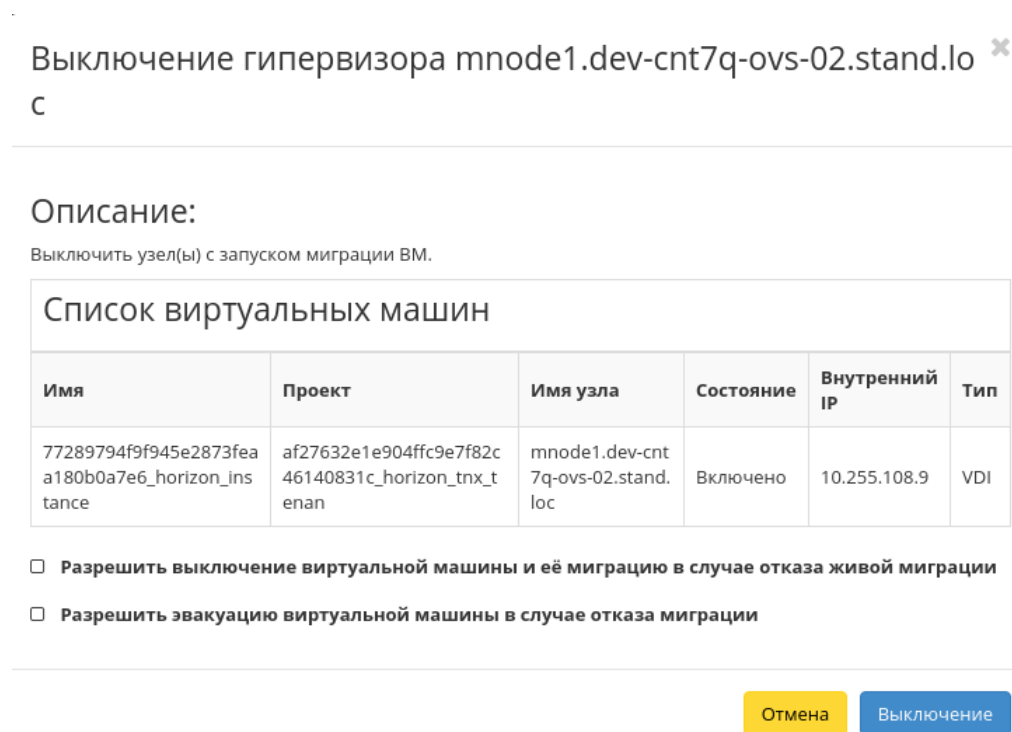
Рис. 4.198: Окно выключения гипервизора
