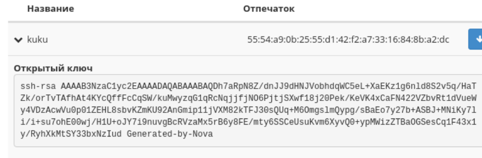
Рис. 4.51: Подробная информация о SSH ключе виртуальной машины
