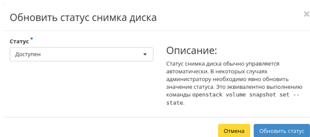
Рис. 4.287: Окно обновления статуса снимка диска
