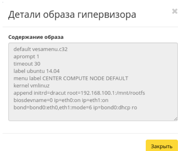
Рис. 4.214: Содержание образа гипервизора
