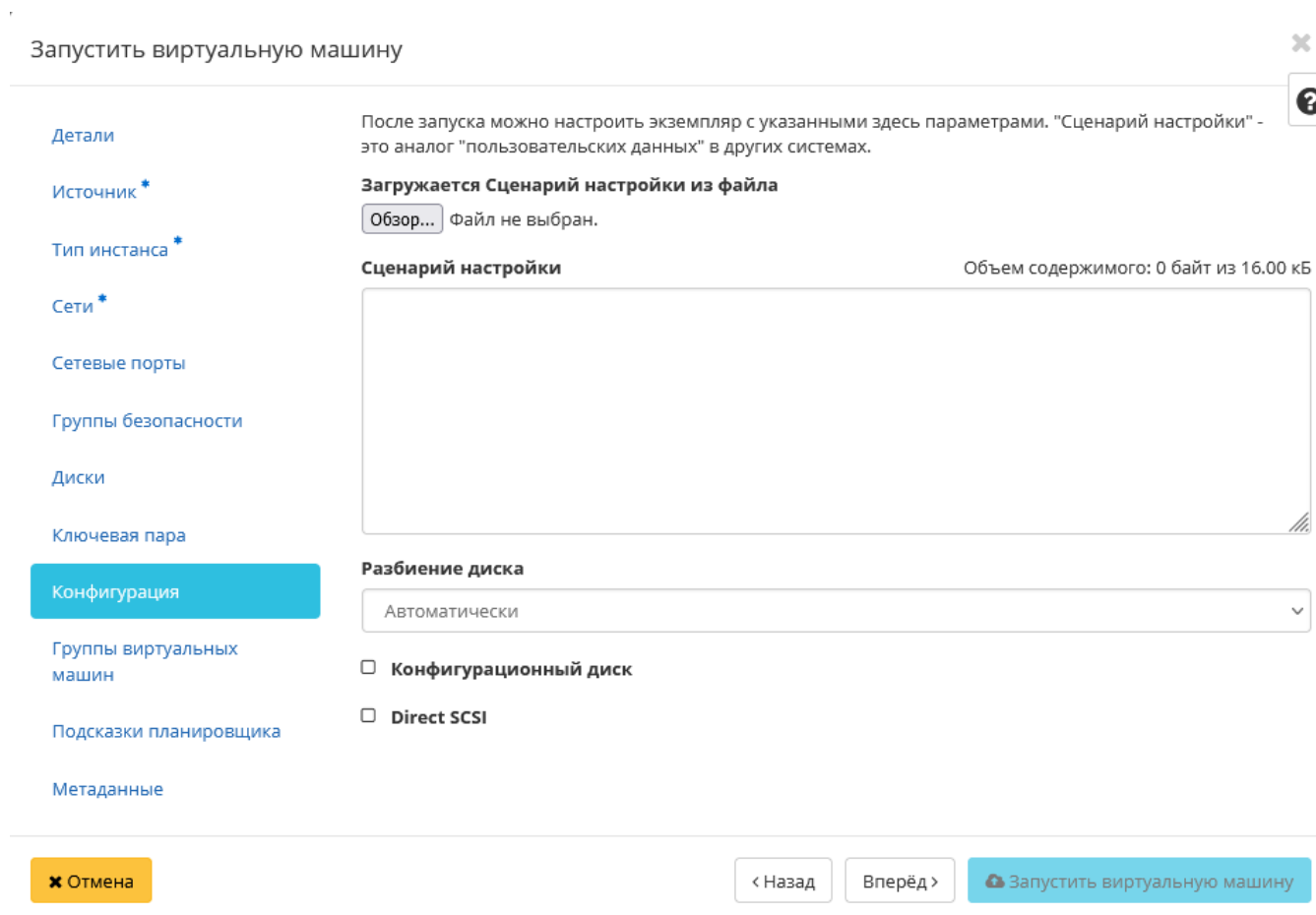
Рис. 4.52: Окно создания виртуальной машины
