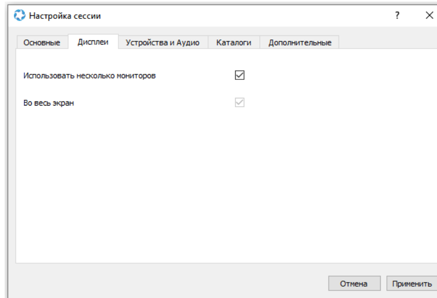
Рис. 3.100: Настройки дисплея VDI-сессии
