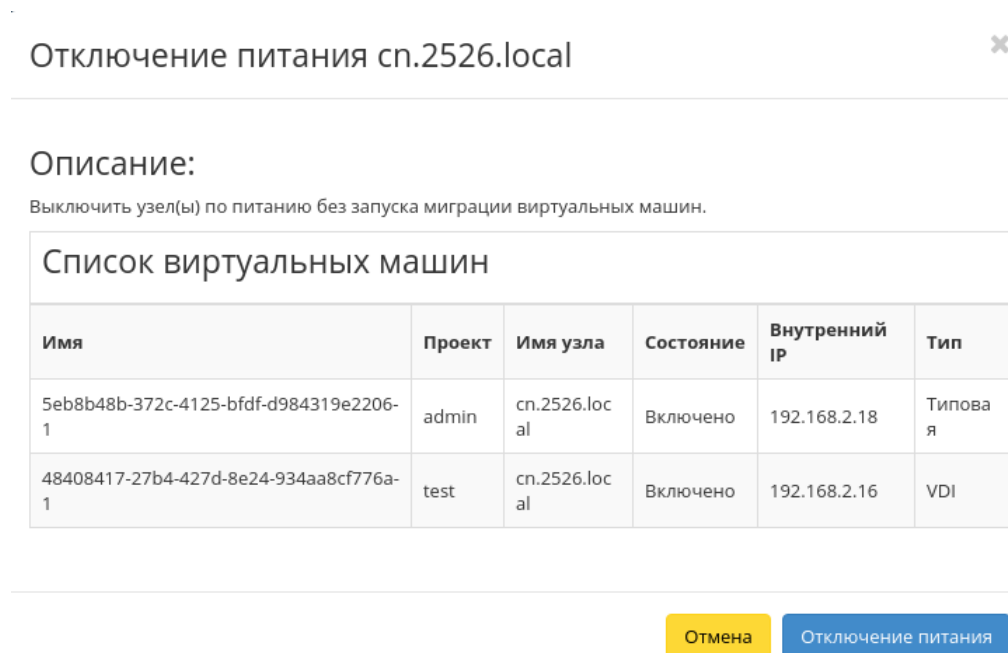
Рис. 4.196: Окно отключения питания гипервизора
